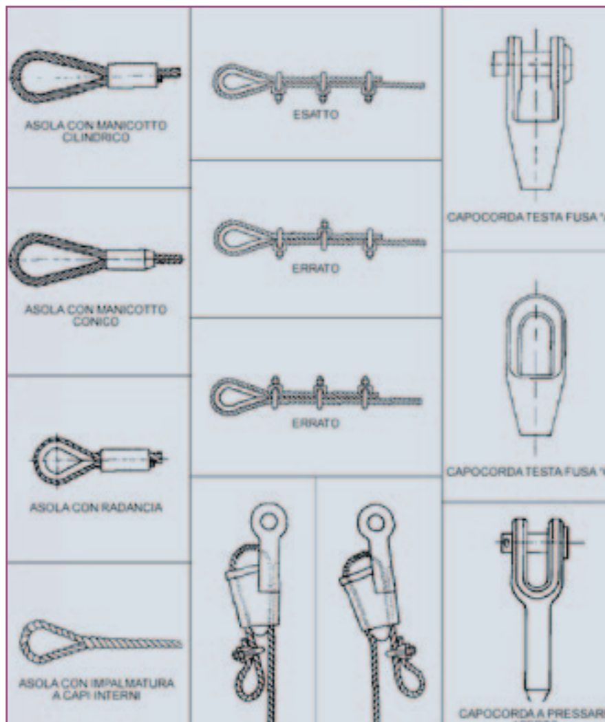
Illustrazione di alcune tipologie di ancoraggio delle funi
